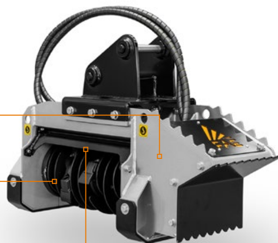
Houe double intégrée au châssis permet de déplacer le matériau à broyer
